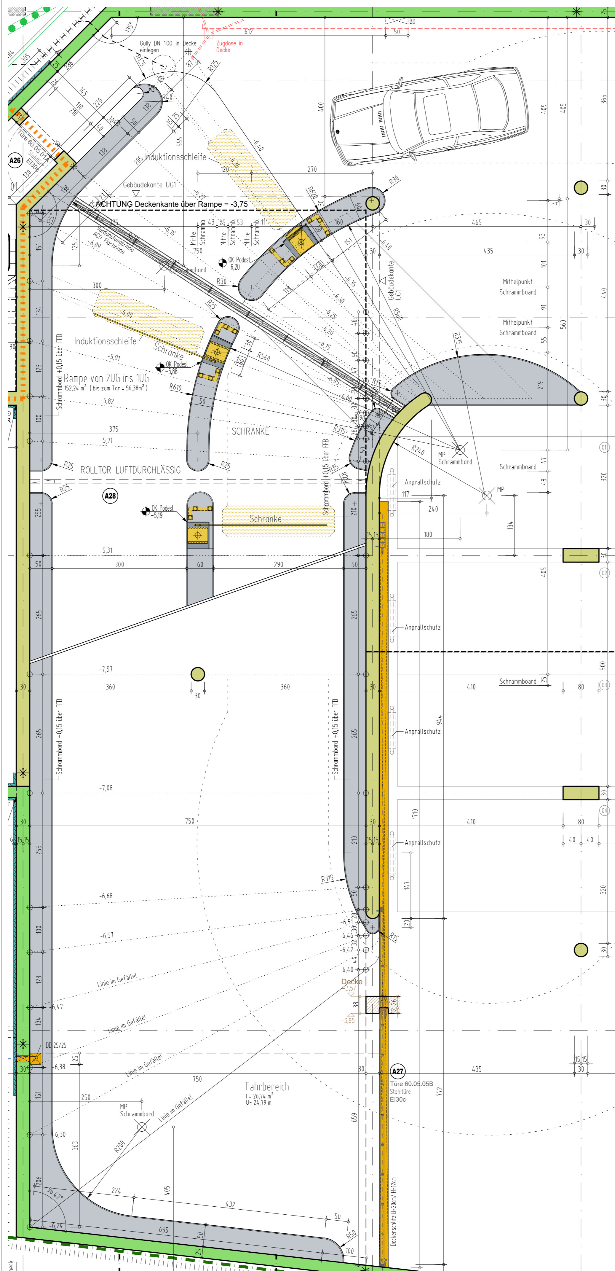
Grundriss UG2
